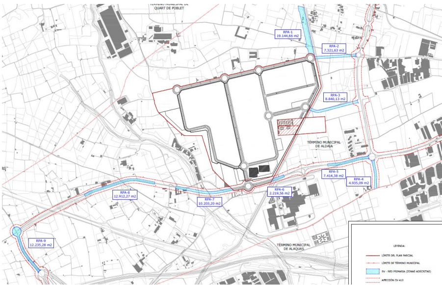
PLANO SECTOR IDENTIFICANDO RED PRIMARIA ADSCRITA
