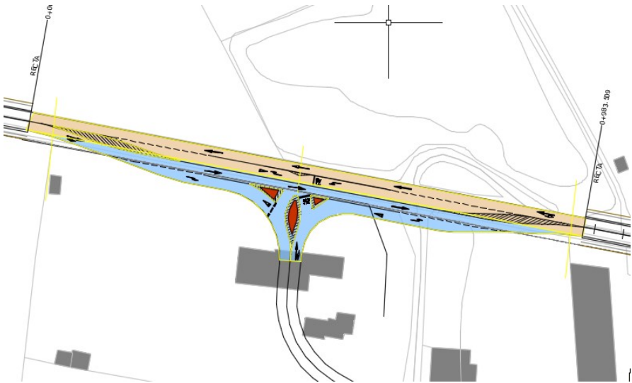
Intersección Beca. Fuente: Elaboración propia.
