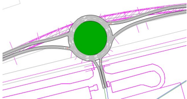
Detalle de GLD desarrollada en AIMSUN
