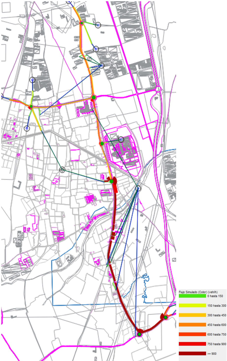
Resultado de flujos en modelo simulado en el Estado Futuro CON Implantación. Fuente: Elaboración propia
