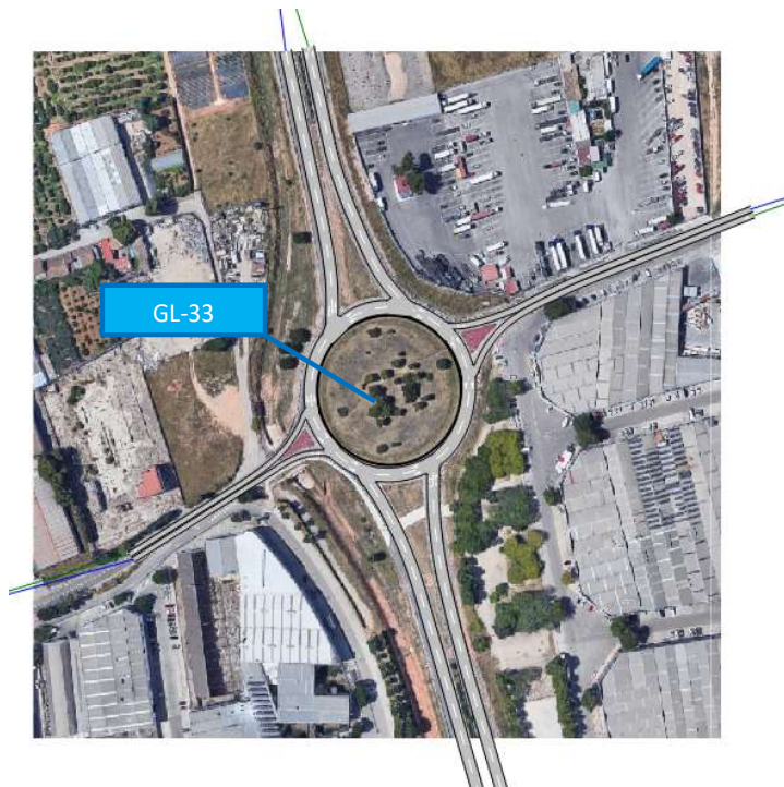
Red simulada Estado Actual. Fuente: Elaboración propia.
