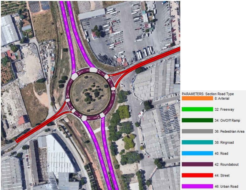
Red simulada Estado Actual / Asignación de características viales. Fuente: Elaboración propia.
