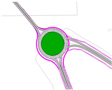
Detalle de GL36 desarrollada en AIMSUN
