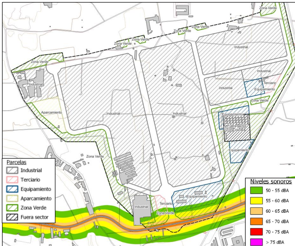
Ilustración 8: Mapa de ruidos L dia actual
