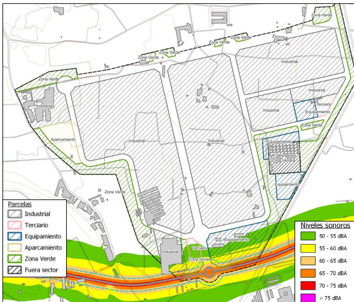
Ilustración 12: Mapa de ruidos Ltarde futuro
