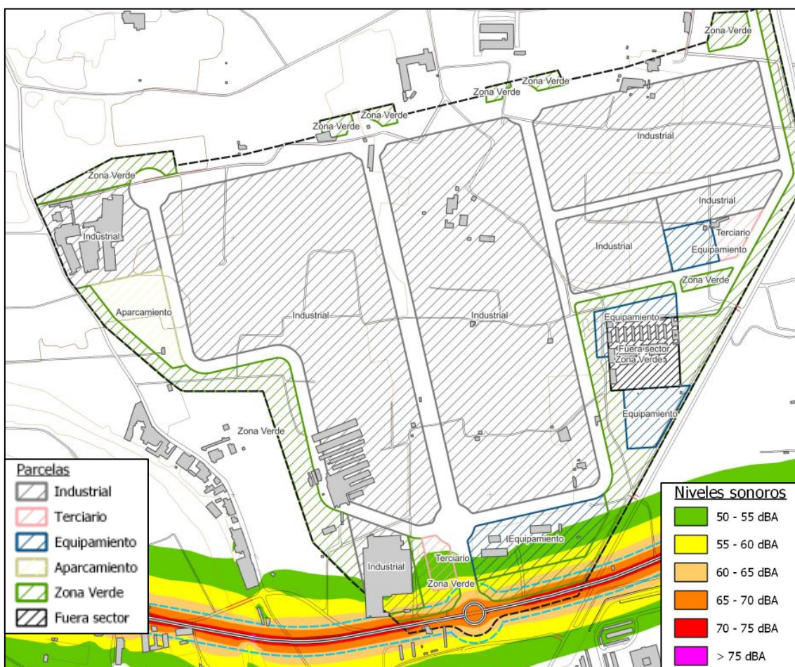
Ilustración 11: Mapa de ruidos Ldía futuro
