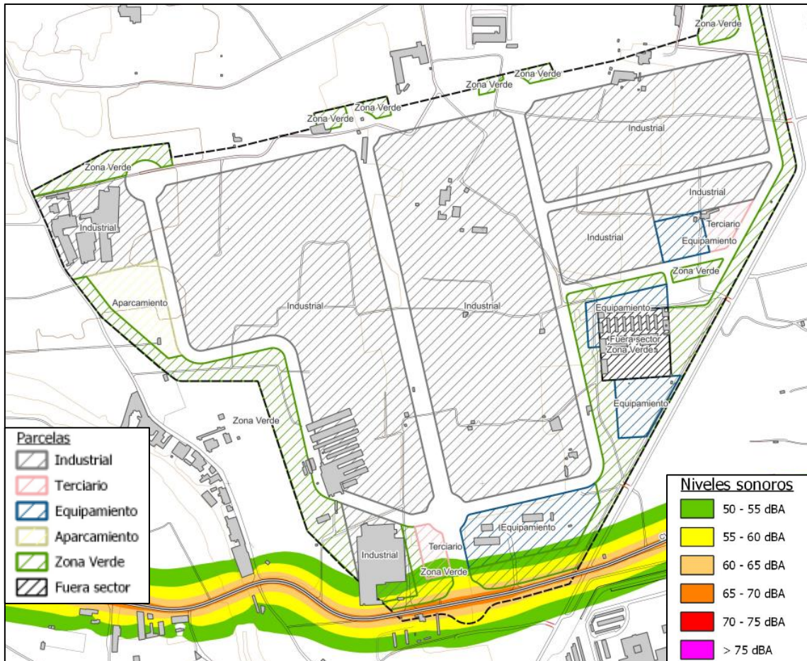
Ilustración 9: Mapa de ruidos Ltarde actual
