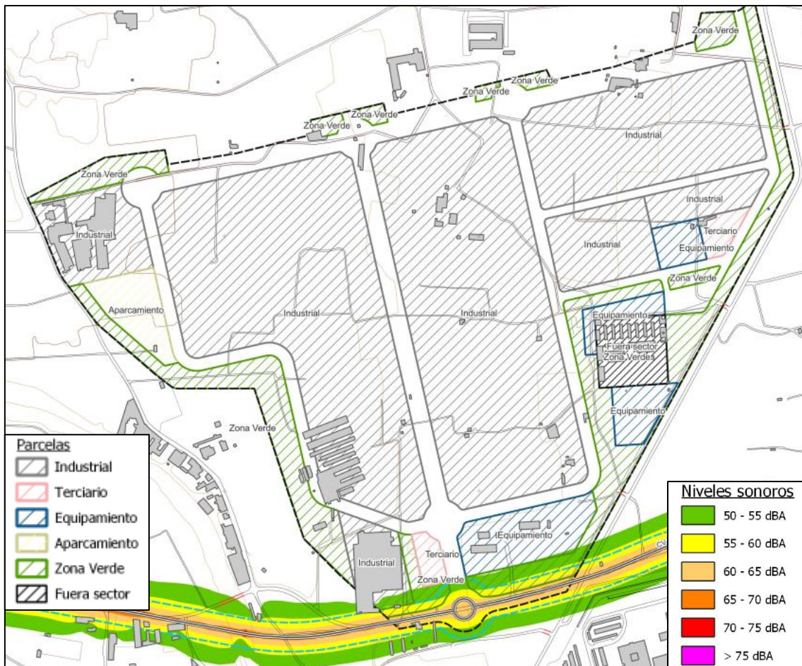
Ilustración 13: Mapa de ruidos Lnoche futuro
