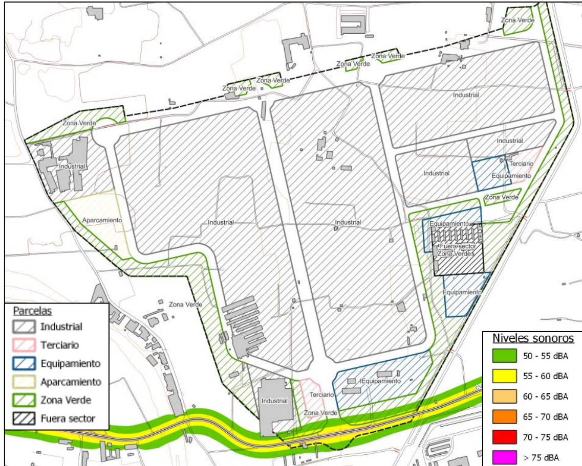
Ilustración 10: Mapa de ruidos Lnoche actual
