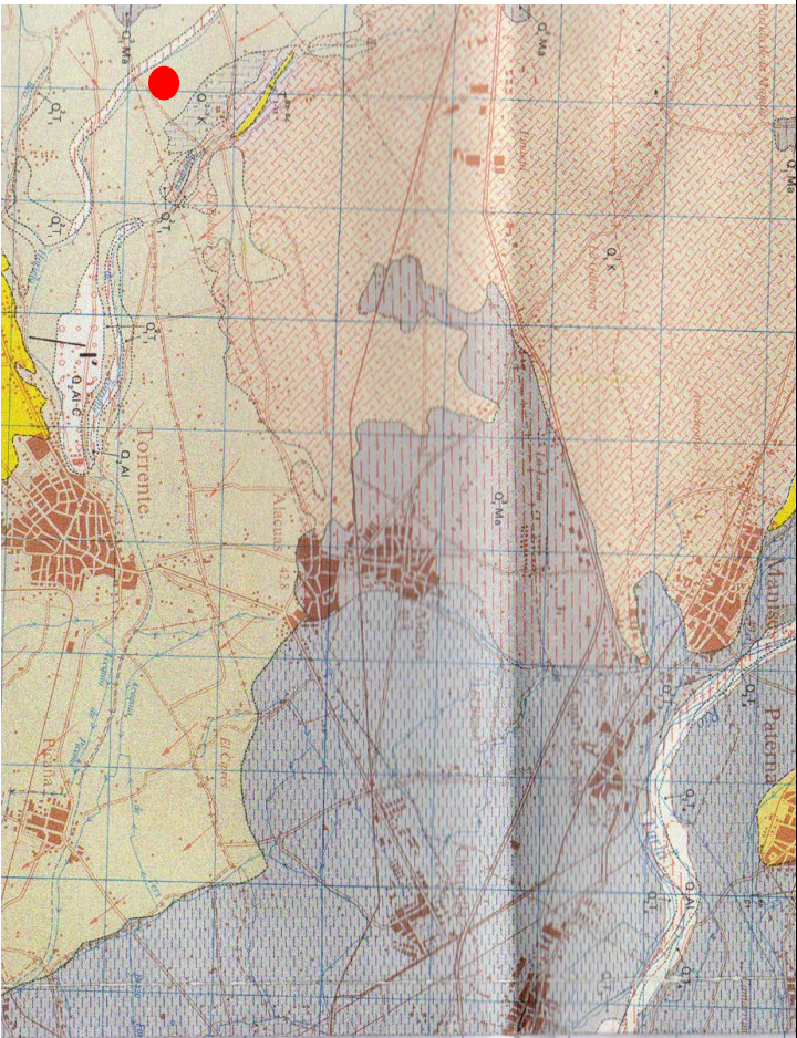
Mapa geológico de la zona de actuación. El círculo señala la zona de la reclasificación pretendida
