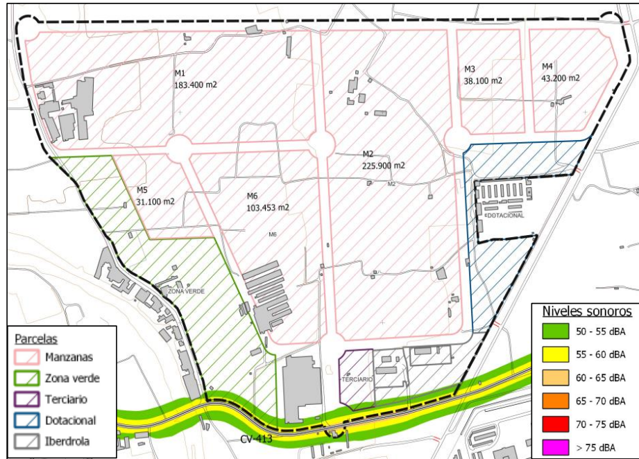
Ilustración 10: Mapa de ruidos Lnoche actual
