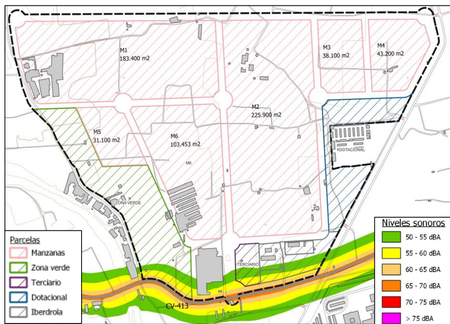
Ilustración 8: Mapa de ruidos Ldia actual
