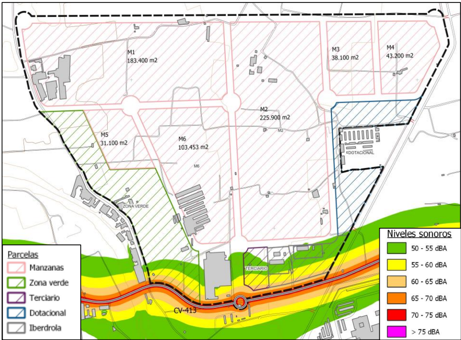
Ilustración 12: Mapa de ruidos Ltarde futuro
