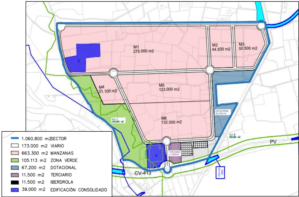
Ilustración 3: Clasificación prevista del suelo
