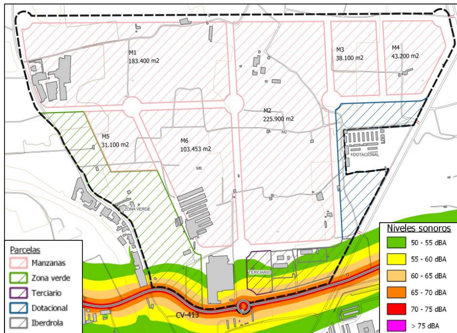
Ilustración 11: Mapa de ruidos Ldia futuro
