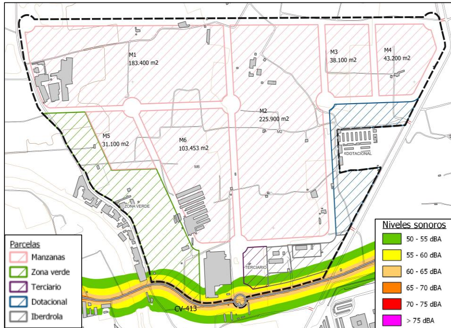
Ilustración 13: Mapa de ruidos Lnoche futuro
